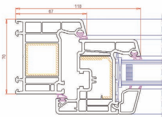
Secção Lateral
