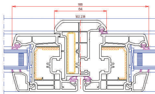
Secção Central
